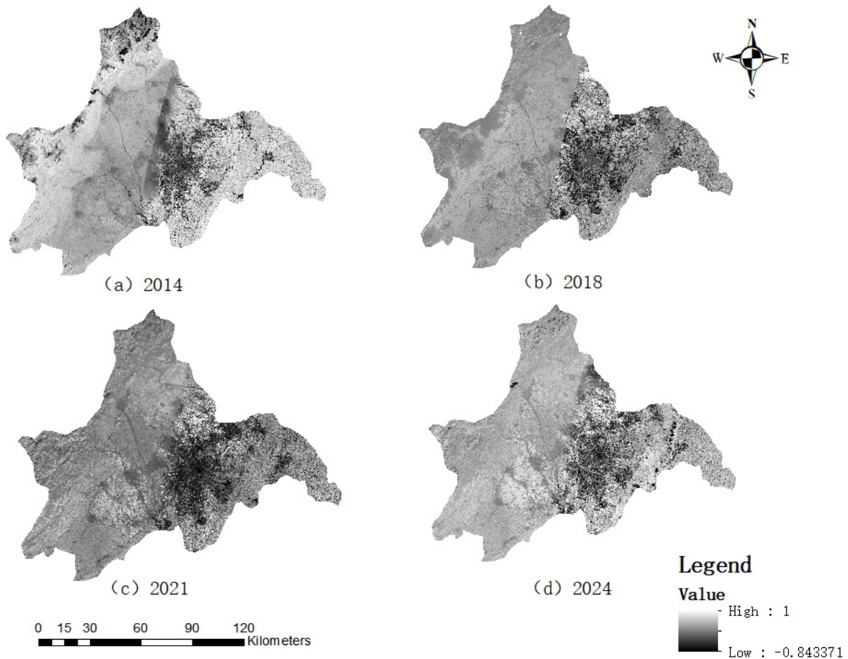
Fig. 2 2014-2024 NDVI images
